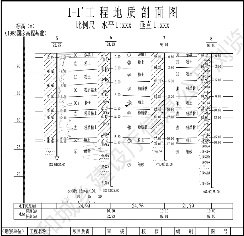
图 B. 1. 2-1 房建工程工程地质剖面图
