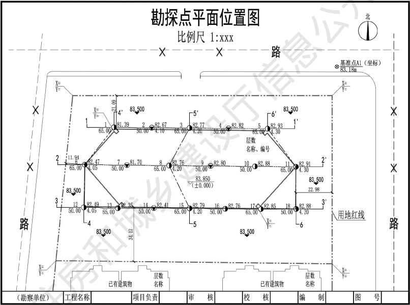
图 B.1.1-1 房建工程勘探点平面位置图
