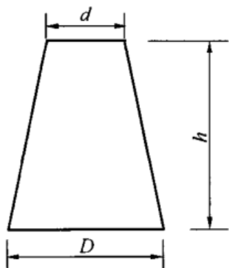
图 A.0.2 砂浆 扩展度筒示意
