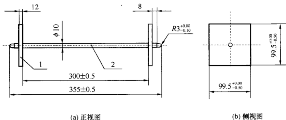
图 B. 0. 2-2 纵向限制器
