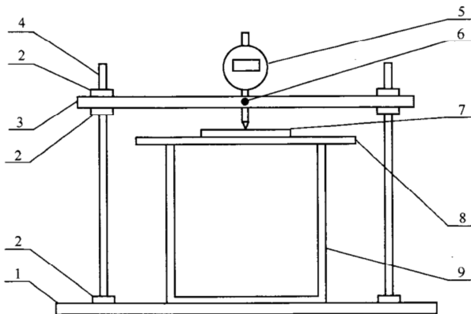
图 C. 0. 3 竖向膨胀率测量装置示意
