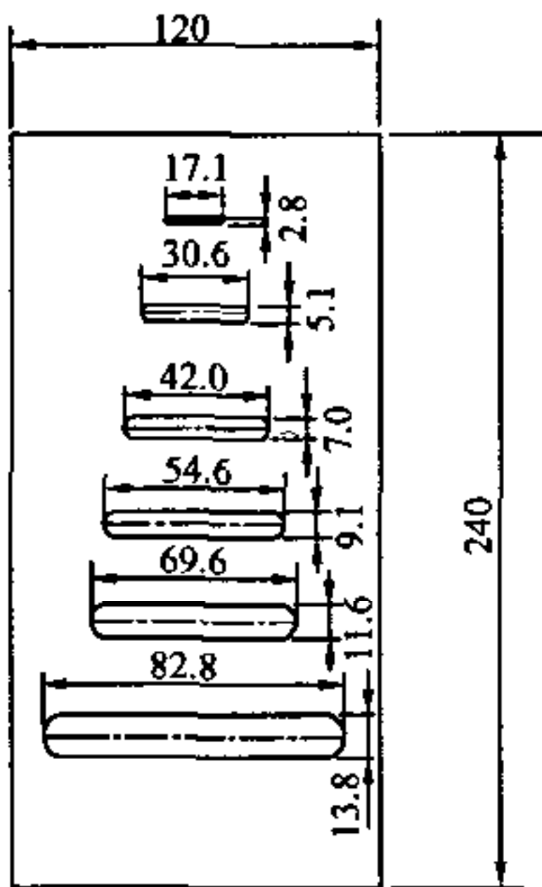
图 7.9.2-2 片状规 准仪 (单位: mm)
