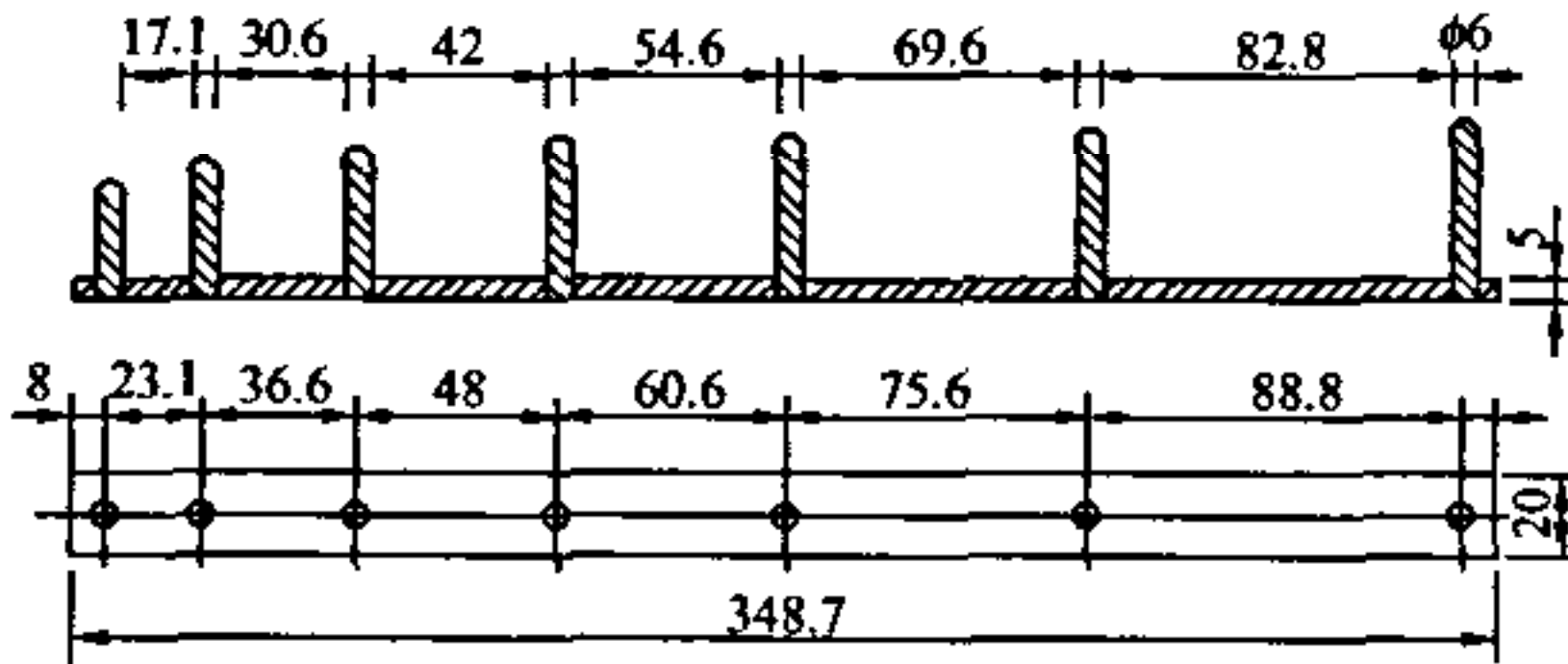
图 7.9.2-1 针状规准仪（单位：mm）
