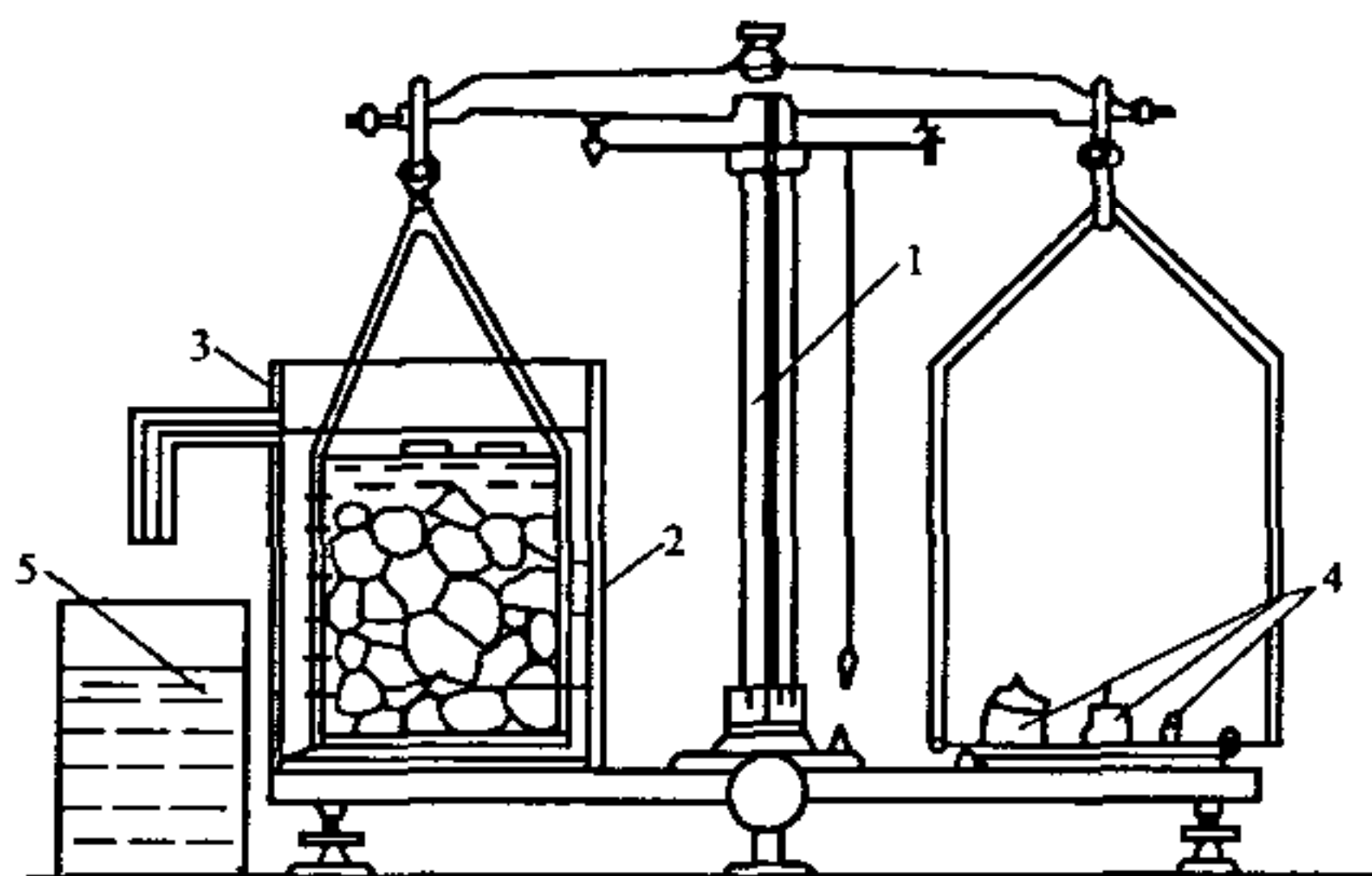
图 7.2.2 液体天平
