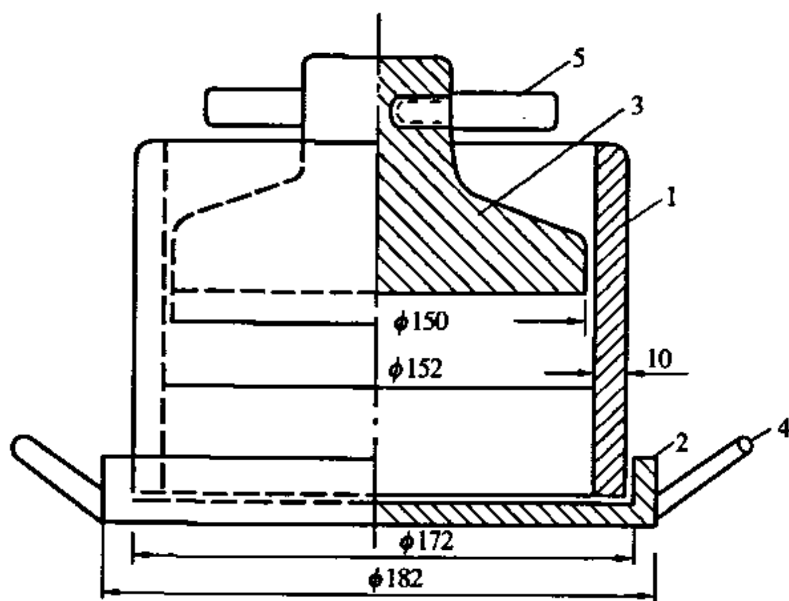
图 7.13.2 压碎值指标测定仪
