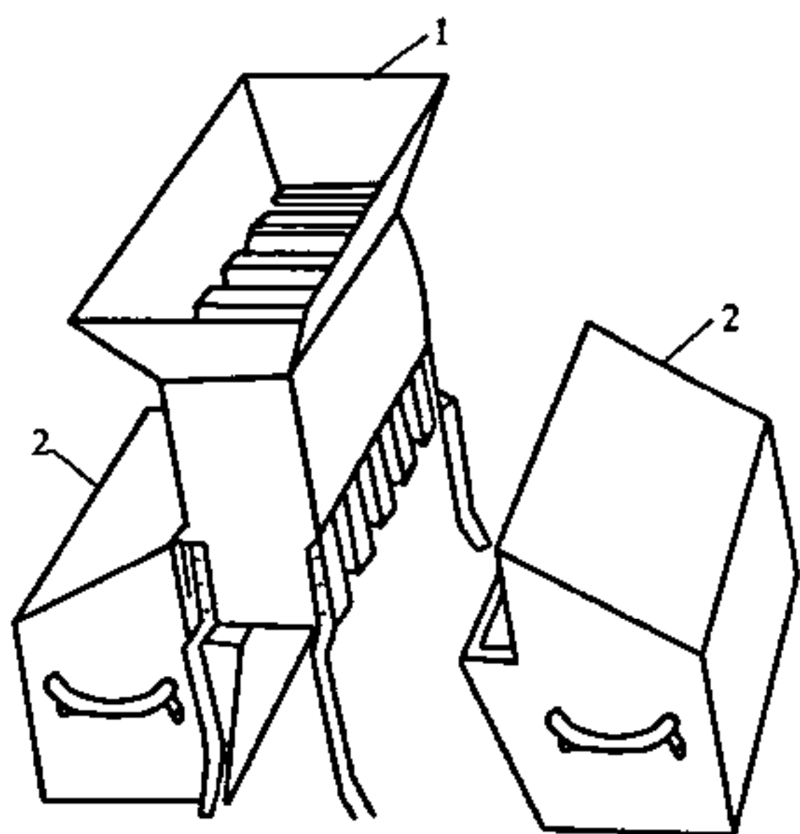
图 5.2.1 分料器 1—分料漏斗；2—接料斗
