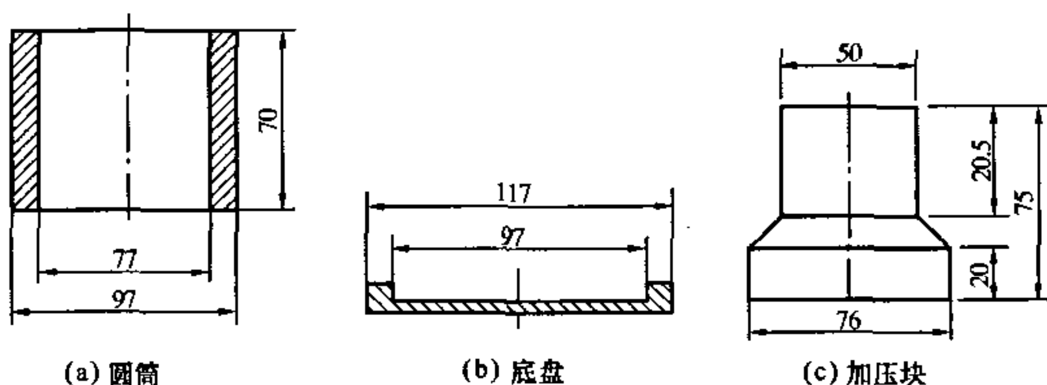
图 6.12.2 受压钢模示意图（单位：mm）
