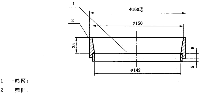
图 1 负压筛
