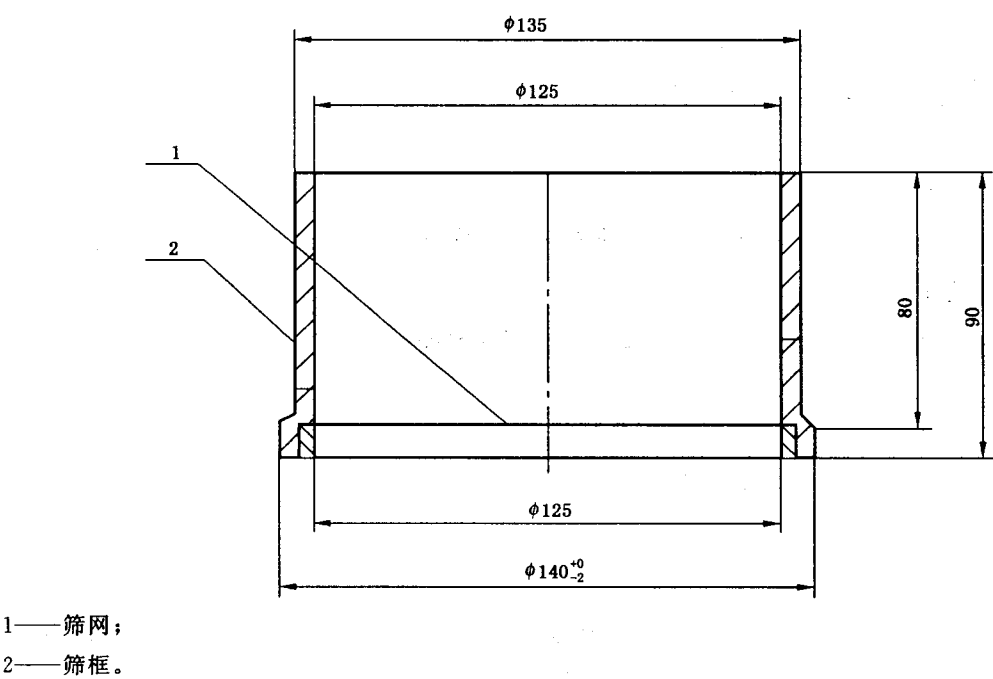
图 2 水筛
