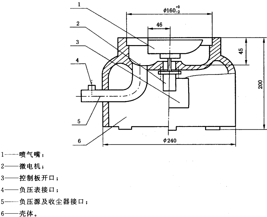
图 3 负压筛析仪筛座示意图
