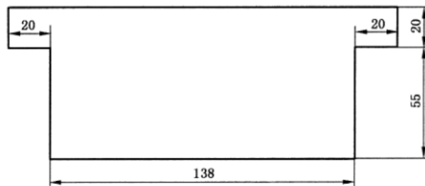
图 2 T 形刮板示意图
